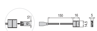
арт.LC11 | Коннектор DC-5050 "мама" 10мм
