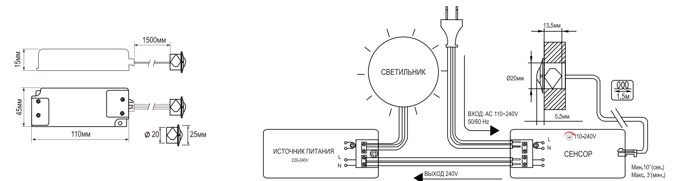
ГАБАРИТНЫЕ РАЗМЕРЫ
