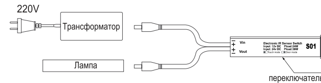
СХЕМА ПОДКЛЮЧЕНИЯ
