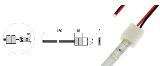
арт.LR24-WP | Коннектор 8мм (2835), IP44
