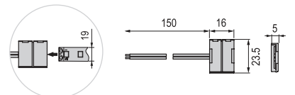
арт.LR33 | Коннектор 19мм (5050-120), IP20
