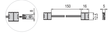
арт.LR21-2 | Коннектор 8мм (2835-120), IP20
