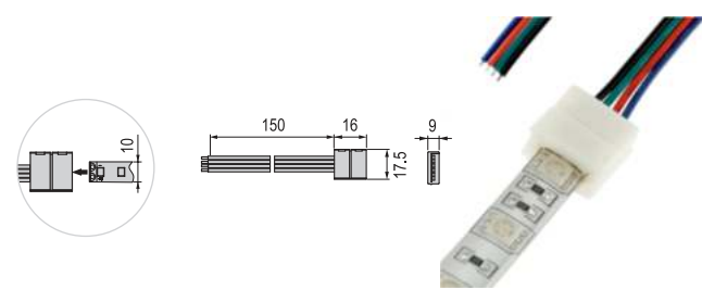
арт.LR26-WP | Коннектор RGB 10мм (5050), IP44
