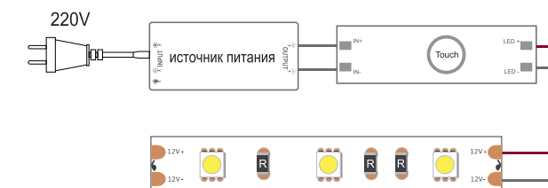
СХЕМА ПОДКЛЮЧЕНИЯ
