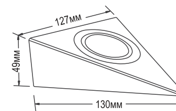
ГАБАРИТНЫЕ РАЗМЕРЫ
