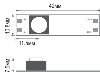
ГАБАРИТНЫЕ РАЗМЕРЫ
