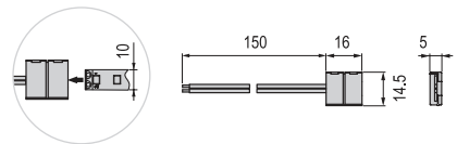
арт.LR25 | Коннектор 10мм (5050), IP20
