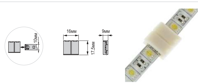
арт.LR28-WP | Коннектор 10мм (5050), IP44
