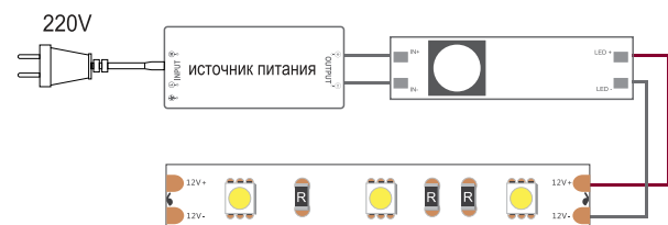
СХЕМА ПОДКЛЮЧЕНИЯ
