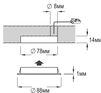
ГАБАРИТНЫЕ РАЗМЕРЫ
