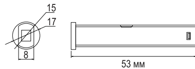
ГАБАРИТНЫЕ РАЗМЕРЫ
