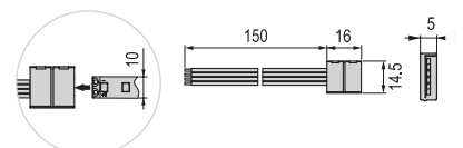
арт.LR26 | Коннектор RGB 10мм (5050), IP20
