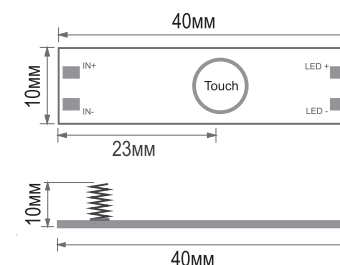
ГАБАРИТНЫЕ РАЗМЕРЫ
