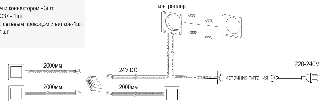
СХЕМА ПОДКЛЮЧЕНИЯ
