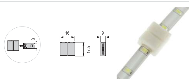
арт.LR27-WP | Коннектор 8мм (2835), IP44
