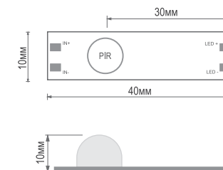
ГАБАРИТНЫЕ РАЗМЕРЫ
