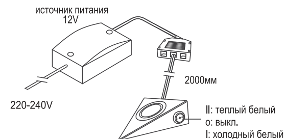
СХЕМА ПОДКЛЮЧЕНИЯ
