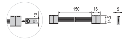
арт.LR23 | Коннектор RGB 10мм (5050), IP20
