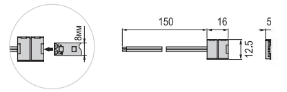
арт.LR24-2 | Коннектор 8мм (2835-120), IP20
