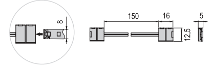
арт.LR21 | Коннектор 8мм (2835-60), IP20
