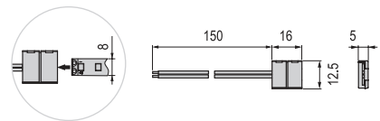
арт.LR24 | Коннектор 8мм (2835-60), IP20
