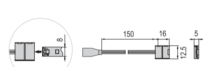
арт.LC10 | Коннектор DC-3528, "мама" 8мм
