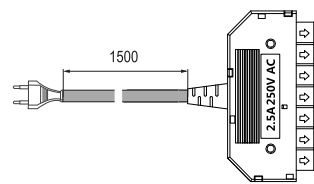
LC-HV06-EU-W | Разветвитель для подключения до 6-и светильников 220V, 2.5А с проводом 1,5м и вилкой EU, IP20
