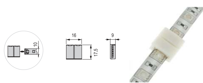
арт.LR29-WP | Коннектор RGB 10мм (5050), IP44
