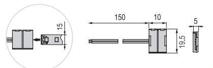
арт.LR32 | Коннектор 15мм (2835-240), IP20
