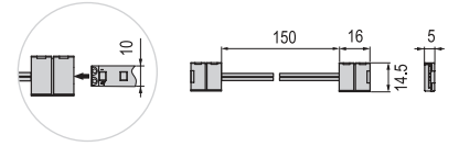
арт.LR22 | Коннектор 10мм (5050), IP20
